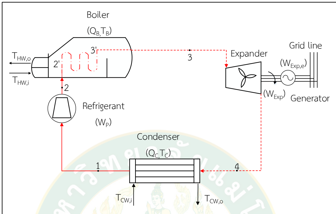
ภาพที่ 10 แผนภาพหลักการทำงานของวัฏจักรแรงดันอินทรีย์
