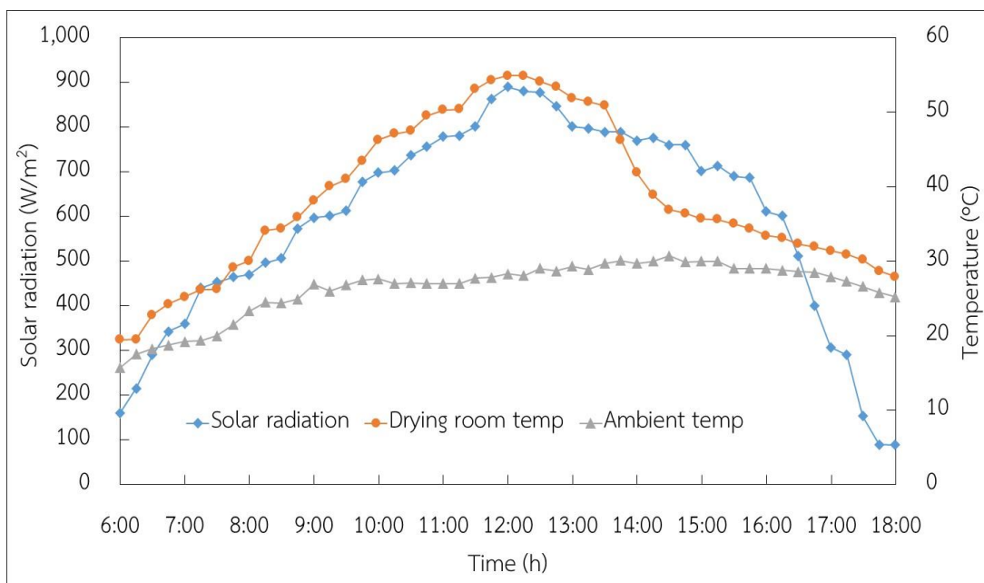
ภาพที่ 35 การตรวจวัดค่ารังสีอาทิตย์อุณหภูมิภายในห้องอบแห้งอุณหภูมิแวดล้อม
