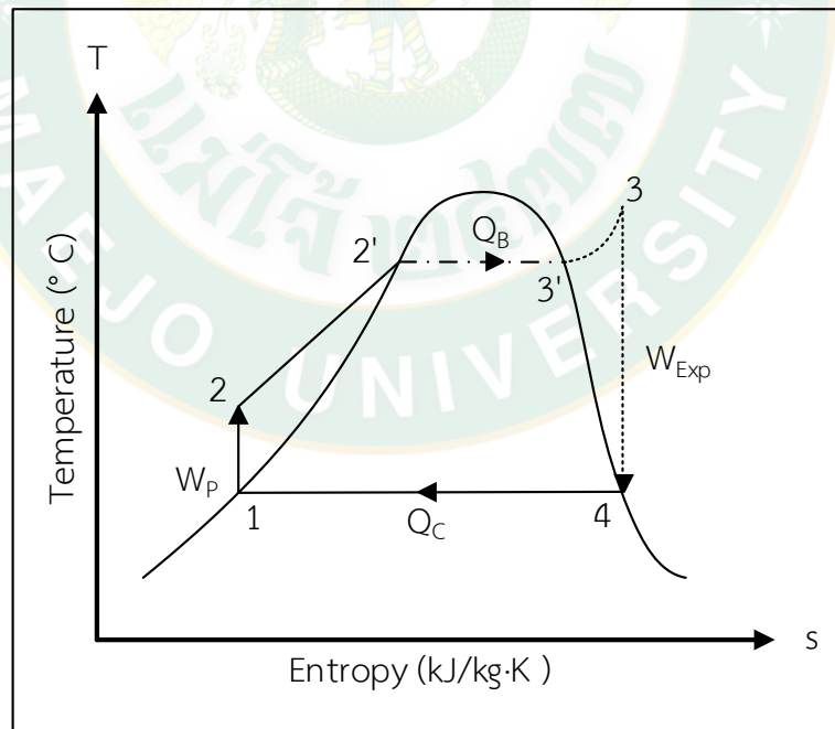
ภาพที่ 11 แผนภาพอุณหภูมิของเอนโทรปี (T-s Diagram) แสดงกระบวนการต่าง ๆ ในแต่ละอุปกรณ์ของวัฏจักรแรงดันอินทรีย์
