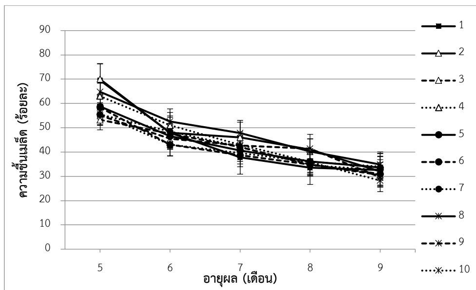
ภาพที่ 4 ผลของสารควบคุมการเจริญเติบโตของพืชต่อร้อยละความชื้นของเมล็ดขนาน้ำมัน ในช่วงอายุผล 5 – 9 เดือน
