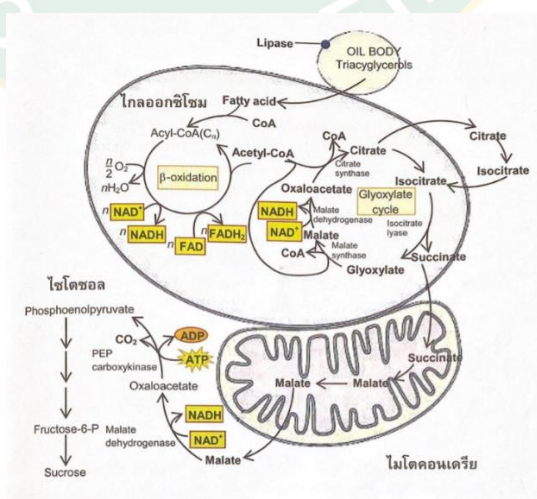
ภาพที่ 2 การสลายกรดไขมัน
