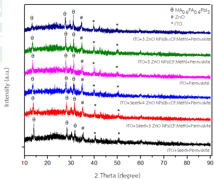
ภาพที่ 55 กราฟ XRD แสดงตำแหน่งของสารเพอร์รอฟสไกต์บนชั้นซิงก์ออกไซด์
