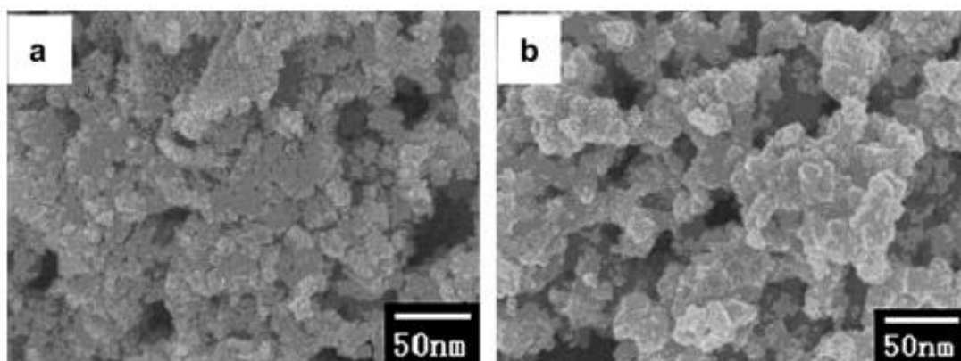
ภาพที่ 40 ภาพ SEM ของอนุภาคนาโนซิงก์ออกไซด์ที่มีการใช้อุณหภูมิที่แตกต่างกัน (a) 80 องศาเซลเซียส (b) 100 องศาเซลเซียส (Liu et al., 2010)
