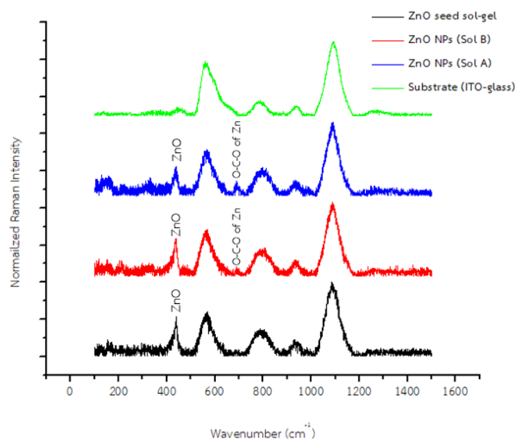
ภาพที่ 53 กราฟแสดงความถี่รามานในช่วงต่างๆ ของซิงก์ออกไซด์ที่นำมาใช้เป็นชั้นนำอิเล็กตรอนใน เซลล์แสงอาทิตย์ชนิดเพอร์รอฟสไกต์
