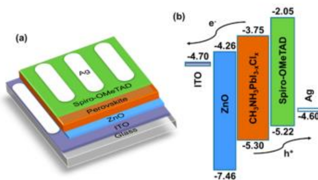
ภาพที่ 29 (a) แสดงโครงสร้างของเซลล์แสงอาทิตย์เพอร์รอฟสไกต์ (b) แสดงชั้นระดับพลังงานของแต่ละชั้น (Zhao et al., 2017)
