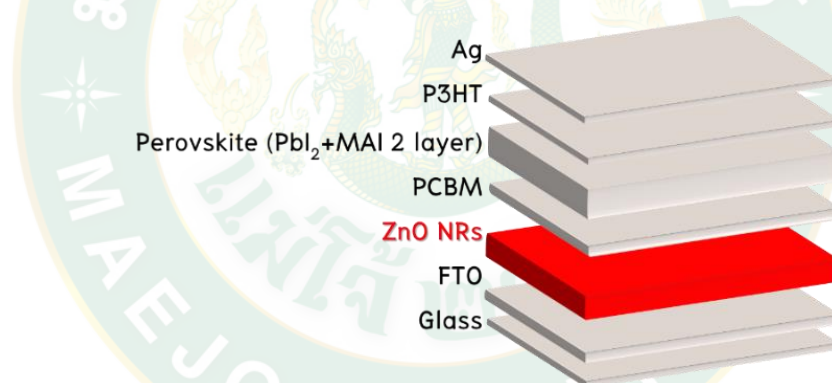
ภาพที่ 43 โครงสร้างที่ใช้โดยมีแท่งนาโนซิงก์ออกไซด์เป็นชั้นนำอิเล็กทรอนิกส์
