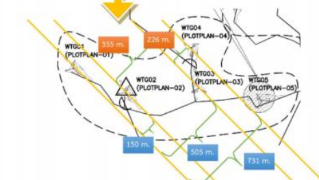
รูปที่ 8 การสร้างเส้นทะแยงมุมบนแผนที่โครงการฯ เพื่อหาระยะห่างระหว่างต้นกังหันตามแนวลม
