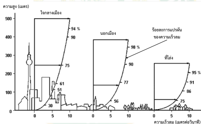
ภาพที่ 15 ผลของความขรุขระของพื้นดินต่อการแปรผันของลม
