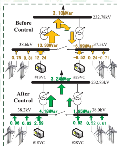
ภาพที่ 25 การควบคุมแรงดันไฟฟ้าของเครื่องกำเนิดไฟฟ้ากังหันลม
