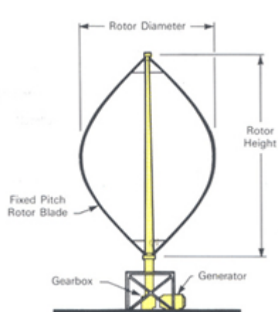
ภาพที่ 6 กังหันลมแบบแนวแกนตั้ง (Vertical axis wind turbine)
