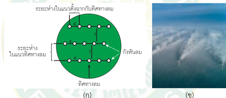
ภาพที่ 16 (ก) ตำแหน่งที่เหมาะสมสำหรับติดตั้งกังหันลม และ (ข) ผลกระทบของความเร็วในทุ่งกังหันลม
