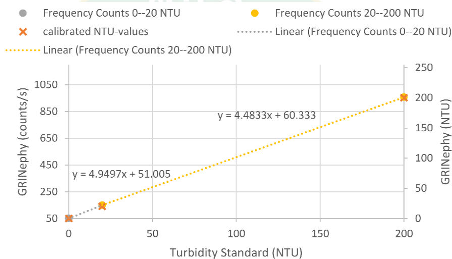
ภาพที่ 7 กราฟมาตรฐานจากการนำค่าที่อ่านได้จากความเข้มข้นของวิธีเนฟิโลเมตริก 0-200 NTU
