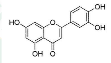
ภาพที่ 5 โครงสร้างของกลุ่มโพลีฟีนอล
