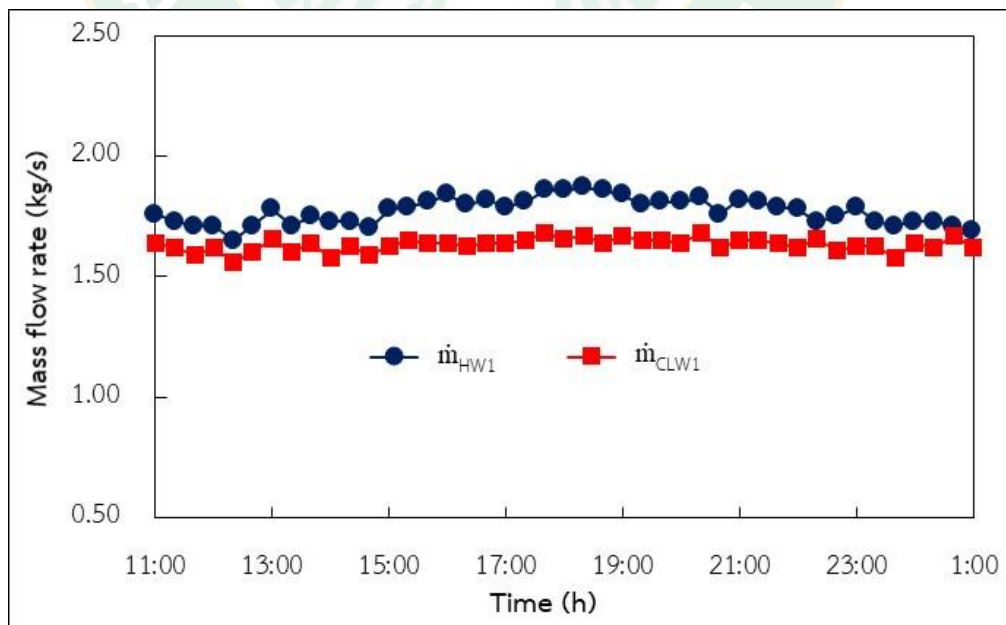
ภาพที่ 49 อัตราการไหลของน้ำร้อนและน้ำหล่อเย็น
