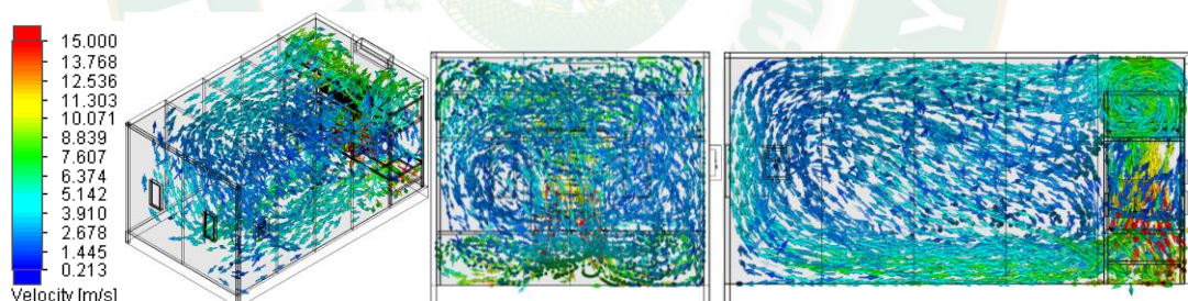
ภาพที่ 41 ลักษณะความเร็วลมของพัดลมแบบหมุนตามแนวแกนขนาดเส้นผ่านศูนย์กลาง 36 in
