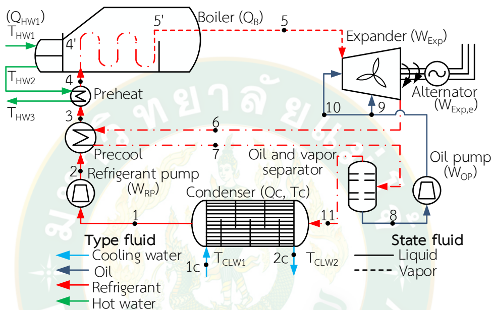
ภาพที่ 3 แผนภาพหลักการทำงานของวัฏจักรแรงดันอินทรีย์
