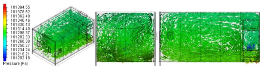
รูปที่ 10 ลักษณะความดันจากพัดลมแบบหมุนตามแนวแกนขนาดเส้นผ่านศูนย์กลาง 20 inch
