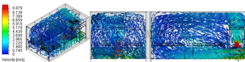
รูปที่ 11 ลักษณะความเร็วลมเมื่อติดตั้งชั้นตะแกรง 1 ชั้น
