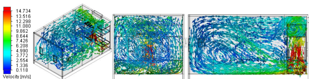
ภาพที่ 40 ลักษณะความเร็วลมของพัดลมแบบหมุนตามแนวแกนขนาดเส้นผ่านศูนย์กลาง 32 in
