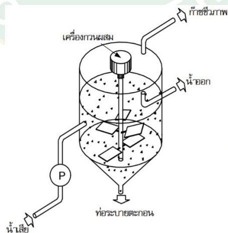
ภาพที่ 7 แผนผังระบบแบบกวนสมบูรณ์
