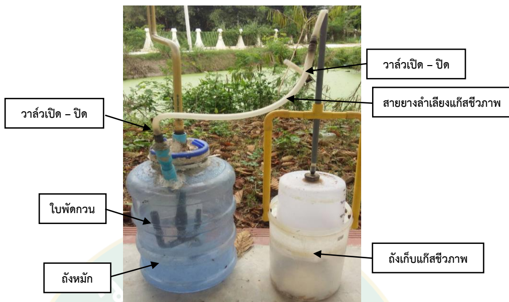
ภาพที่ 21 การทดลองผลิตแก๊สชีวภาพในระดับห้องปฏิบัติการ
