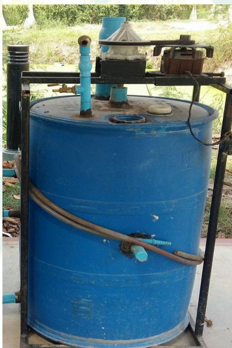
ภาพที่ ค-2 ชุดถังหมักแก๊สชีวภาพระดับครัวเรือน
