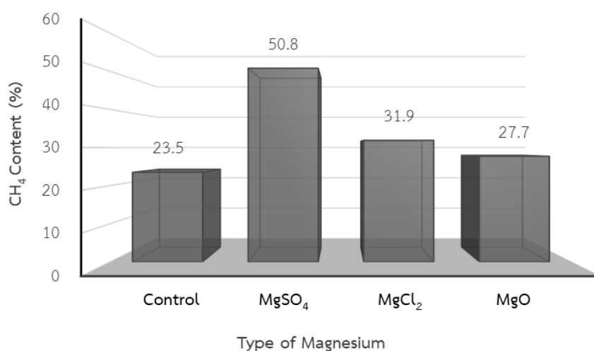
ภาพที่ 27 ผลขององค์ประกอบแก๊สมีเทนในกระบวนการหมักหลังผ่านการตกตะกอนโดยใช้สารประกอบแมกนีเซียม
