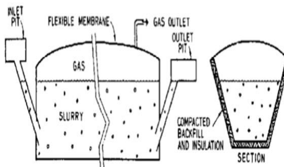
ภาพที่ 4 บ่อหมักข้าวแบบราง
